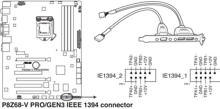
P8Z68-V PRO/GEN3 IEEE 1394 connector
