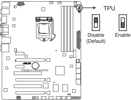
P8Z68-V PRO/GEN3 TPU switch
